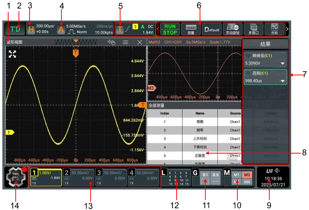
图 4.5 用户界面
