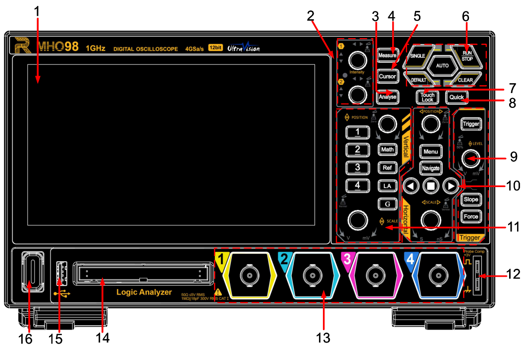
图 4.3 前面板
