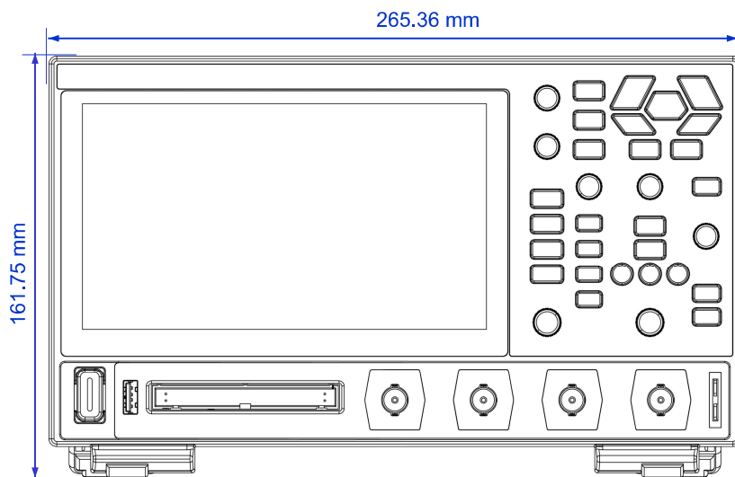
图 4.1 正视图
