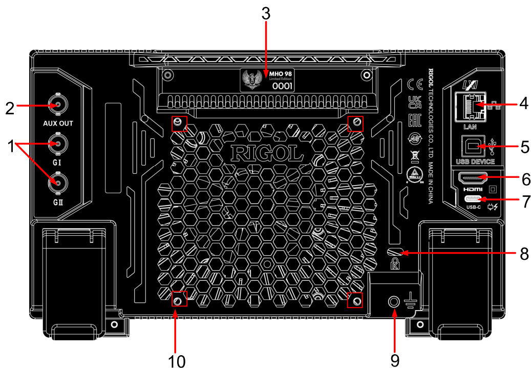
图 4.4 后面板
