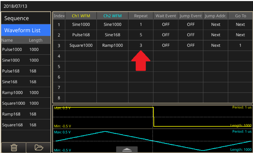
图 100：设置重复函数
