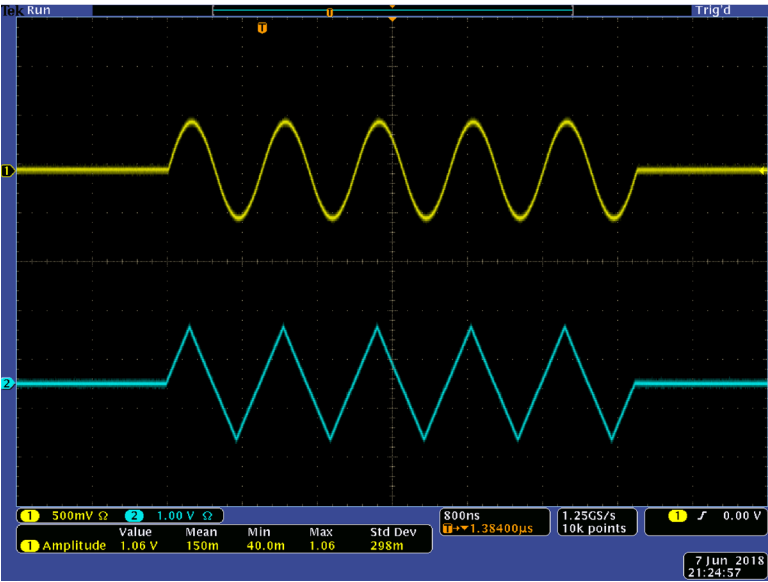
图 61：同步后的主从仪器
