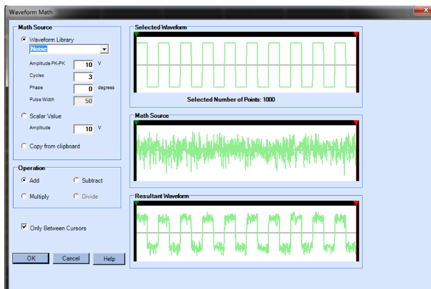
图 159: ArbExpress 数学应用程序
