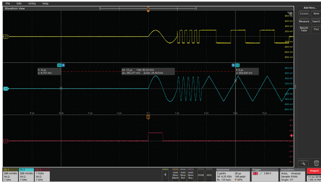
图 110：单触发波形
