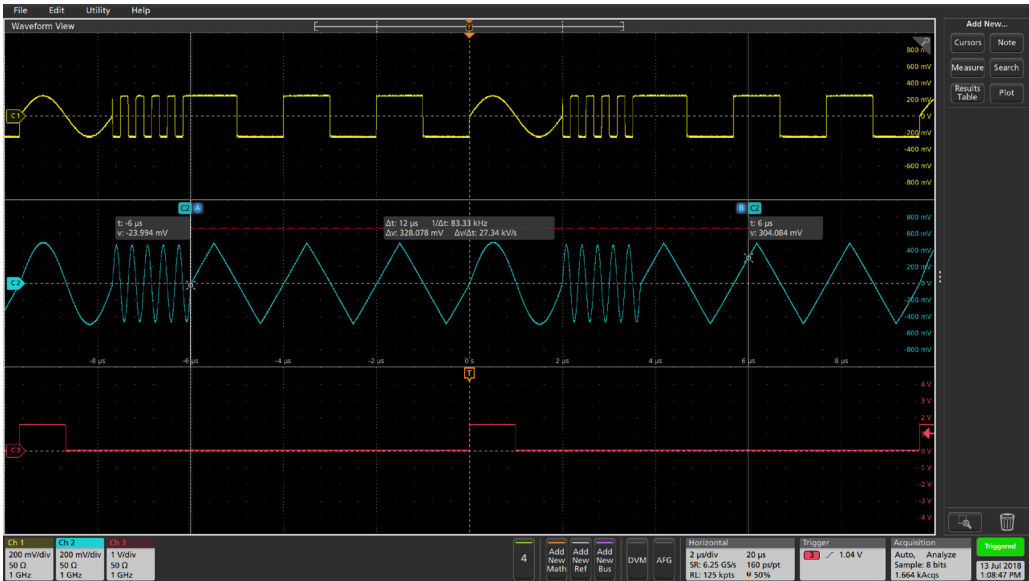
图 106: 观察示波器的变化
