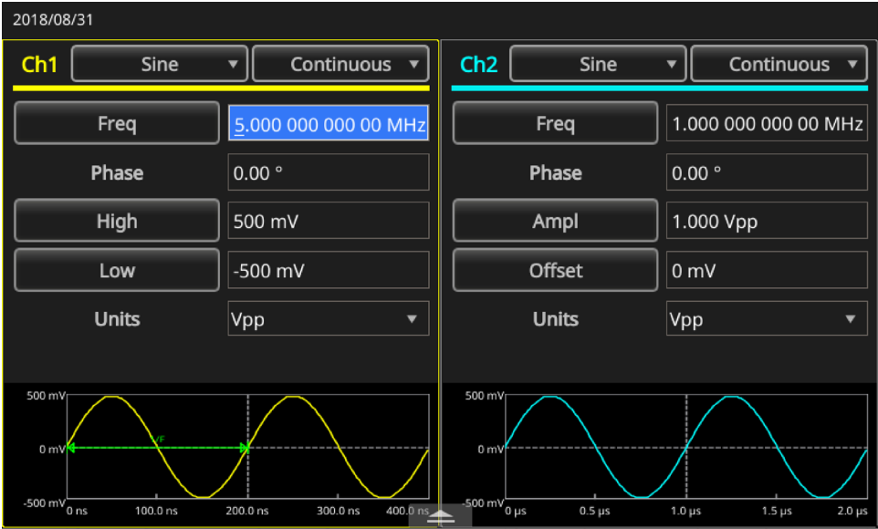
图 43：CH1 频率 5 MHz
