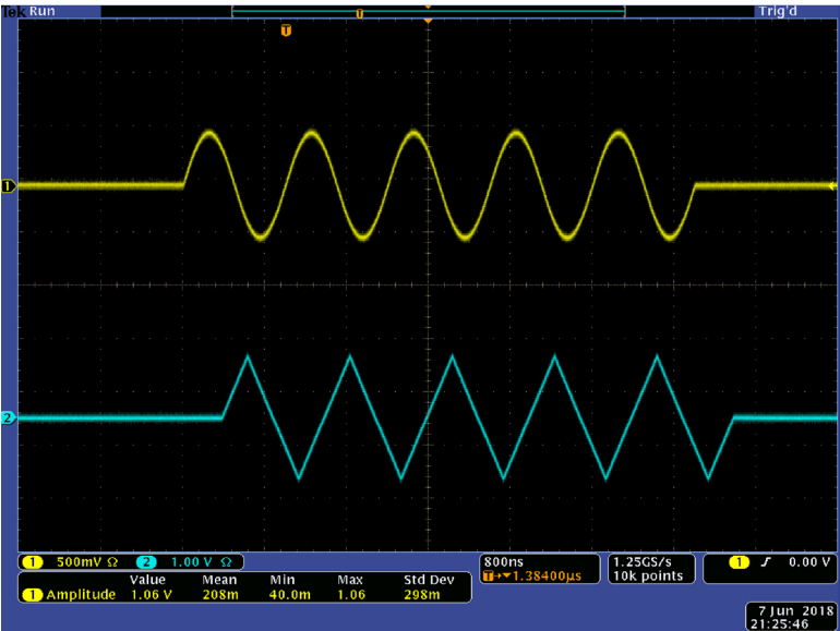
图 60：同步前的主从仪器
