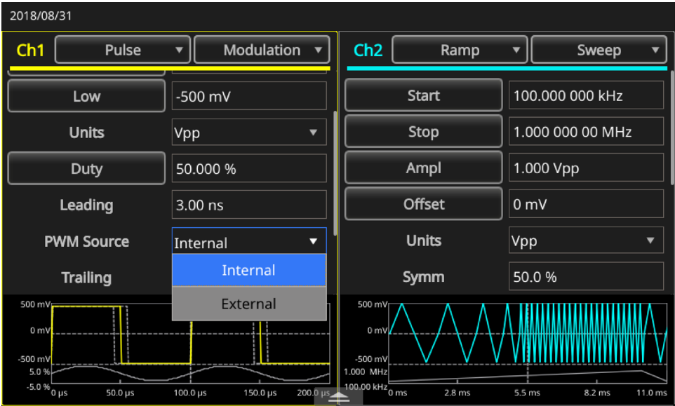
图 40：PWM 信号源设置
