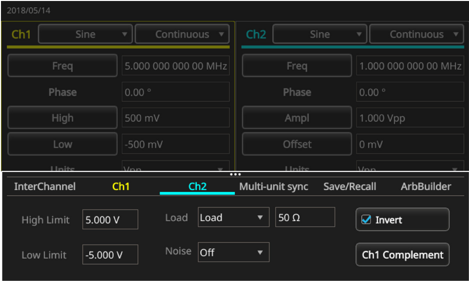
图 53：CH2 选项卡和 CH1 补充按钮
