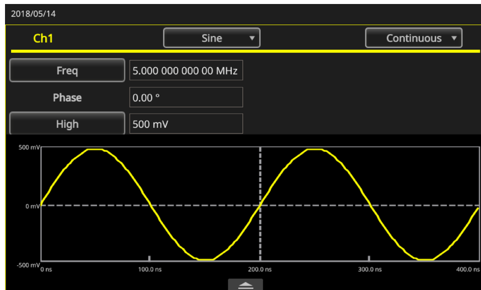
图 48：无噪声
