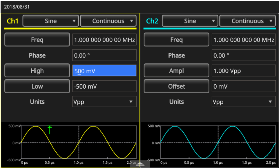
图 8：高位按钮为有效状态
