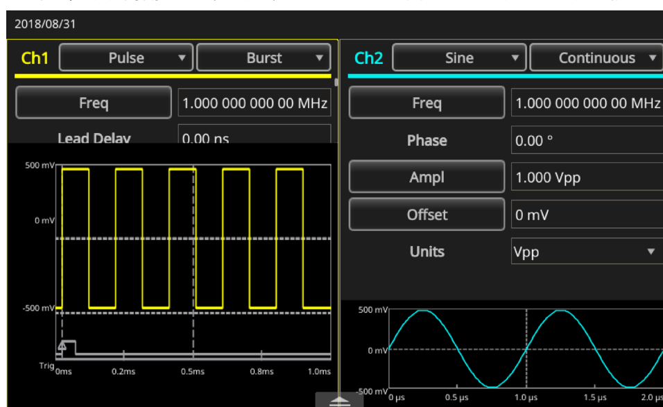
图 31：突发脉冲波形
