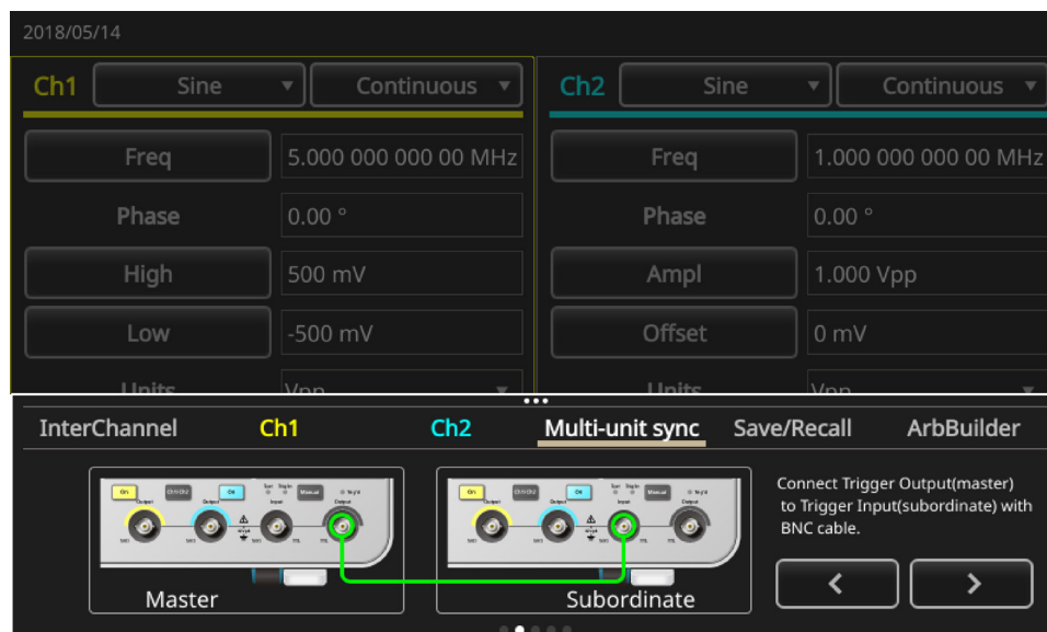
图 55: “多同步仪器” 选项卡 2
