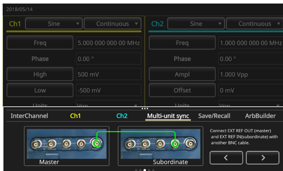
图 56: “多设备同步” 标签 3
