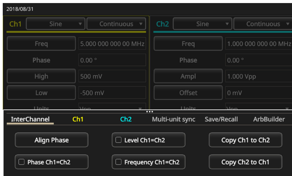
图 44：校准 CH1 和 CH2
