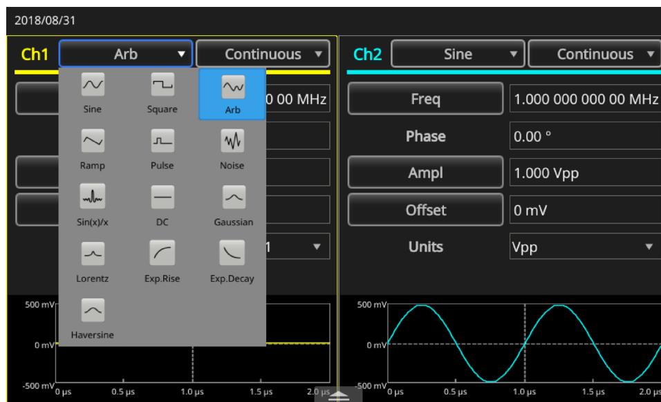
图 13：选择 Arb 波形
