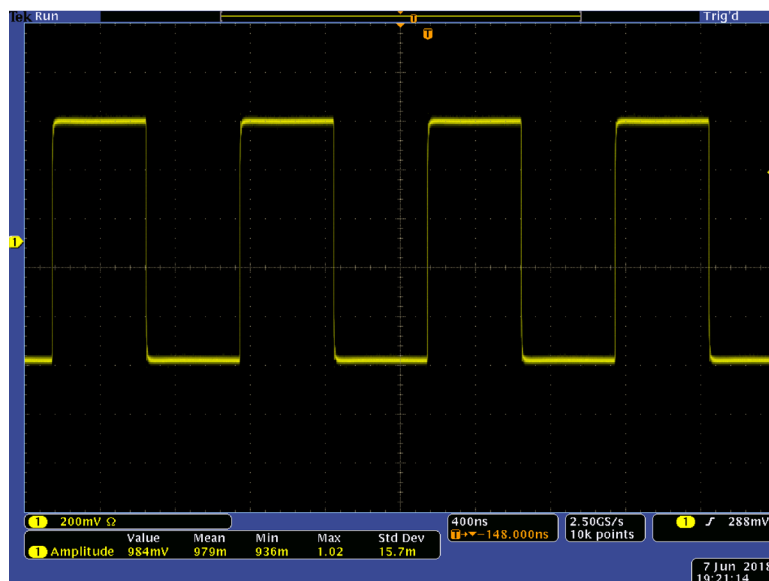
图 50：噪声前的外部信号
