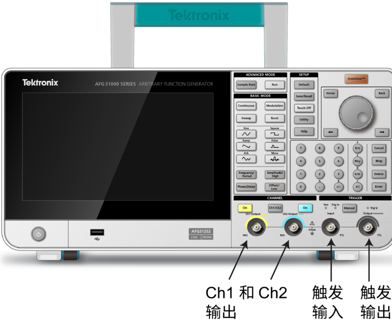
图 2：AFG31000 系列前面板输入和输出
