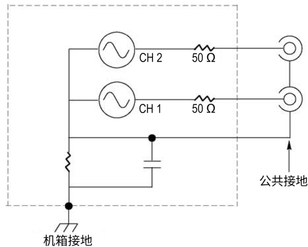
图 3：AFG31000 系列浮动接地
