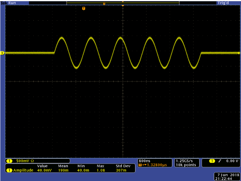
图 59：主仪器波形
