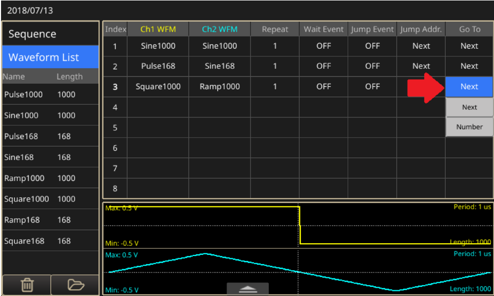
图 98：“转到”字段，更改为 1
