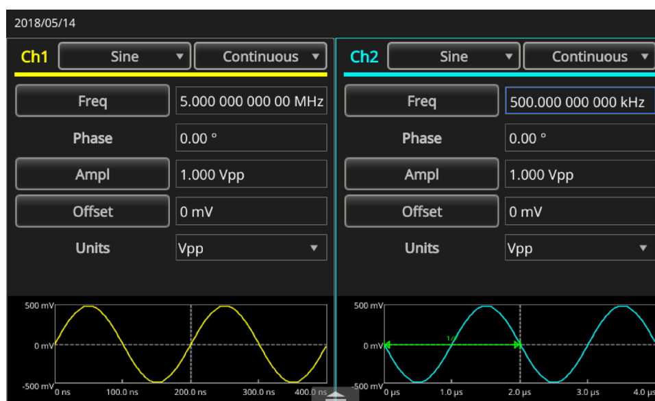
图 161：设置波形码型
