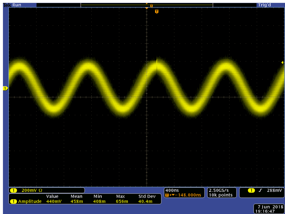
图 49：添加噪声之后的波形
