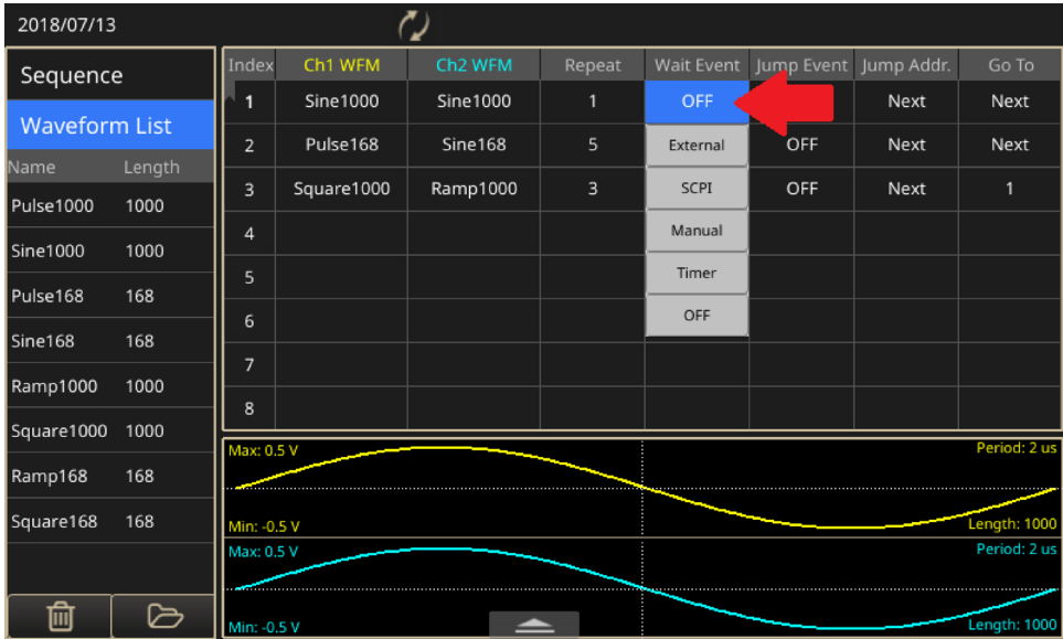
图 107: Wait Event - 序列
