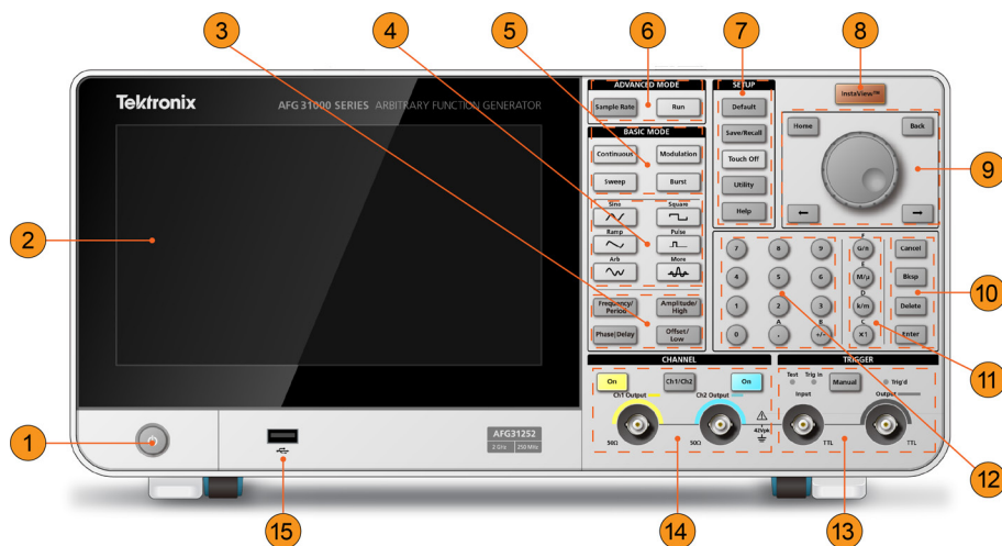
图 6：AFG31000 系列仪器前面板概述
