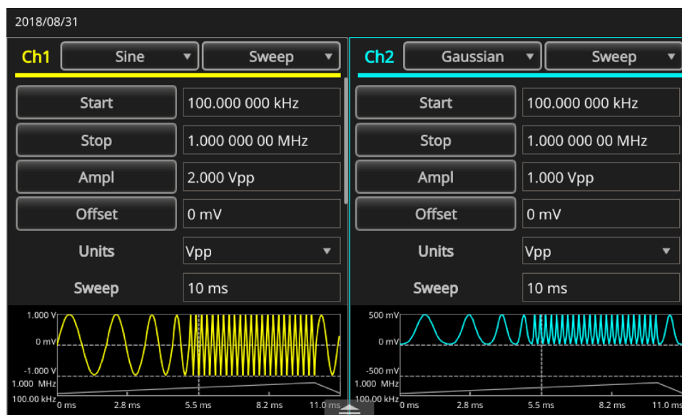
图 33：扫描波形设置
