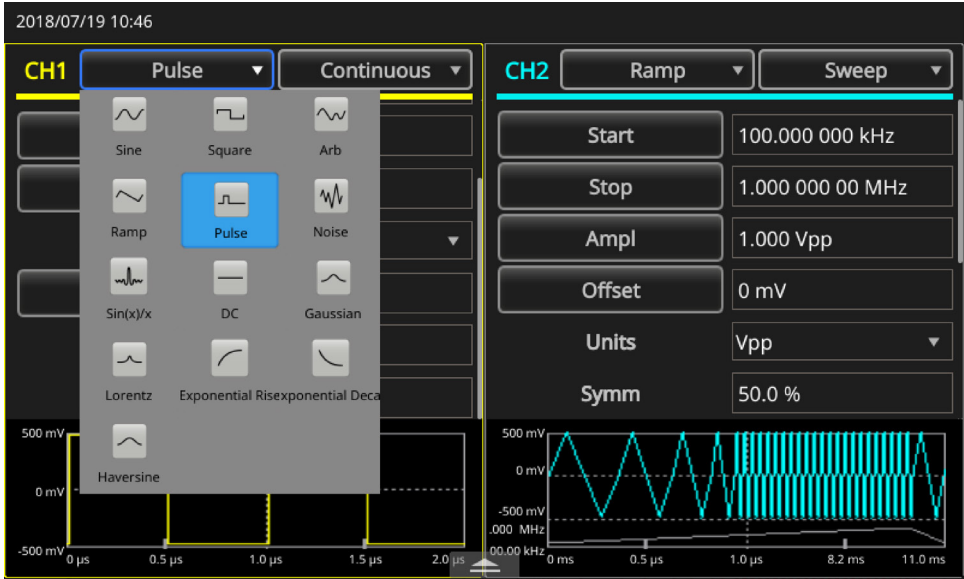
图 38：选择脉冲
