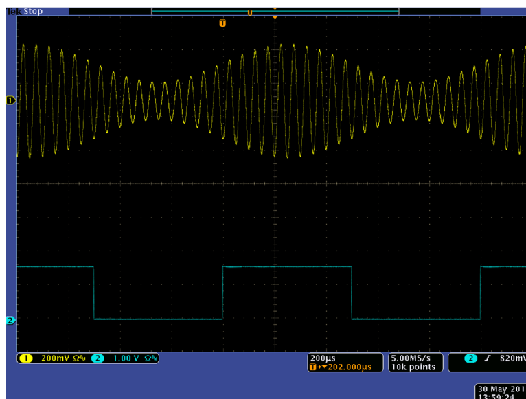
图 35：示波器幅度调制波形
