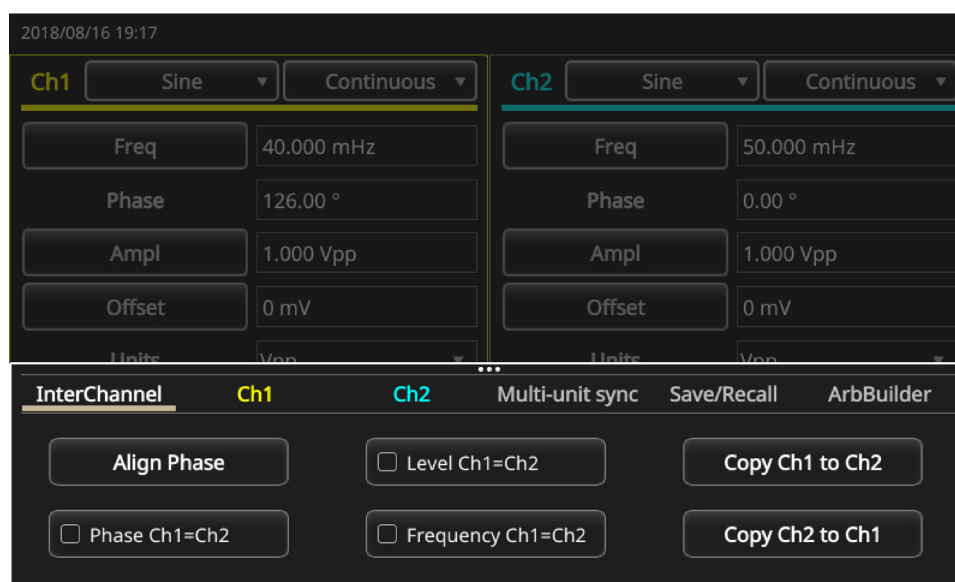
图 45：将通道 1 复制到通道 2
