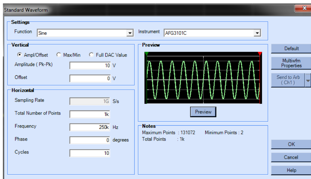
图 157: ArbExpress 标准波形
