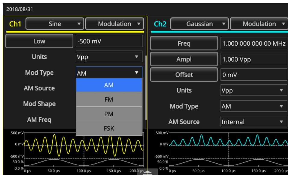
图 37：调制类型
