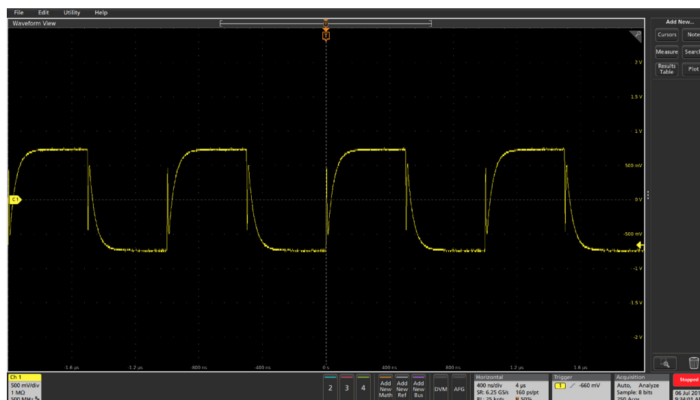
图 74: 复合负载
