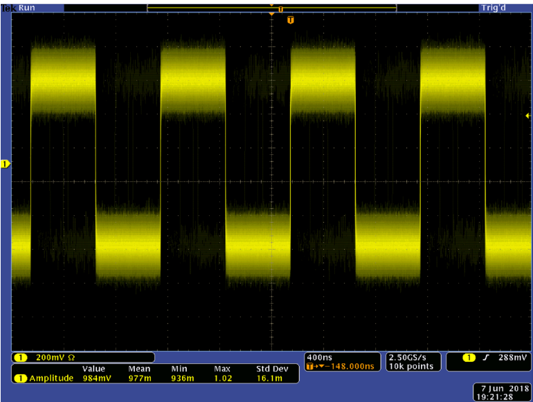
图 51：噪声后的外部信号
