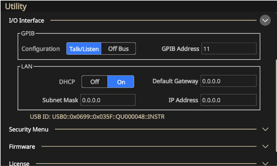
图 121：I/O 接口选项
