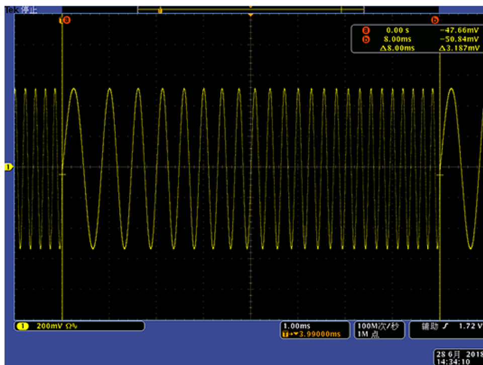
图 167：测量频率特性
