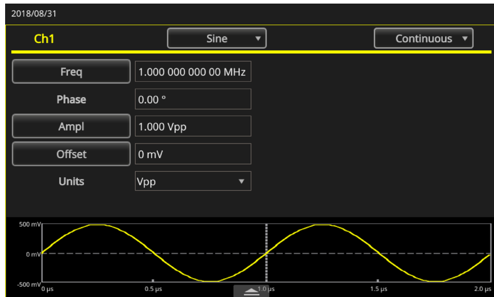
图 21：单通道 AFG 主屏幕
