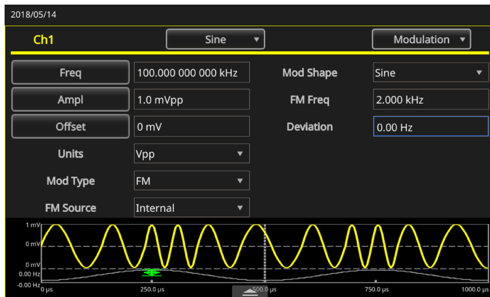
图 170：载波波形频率
