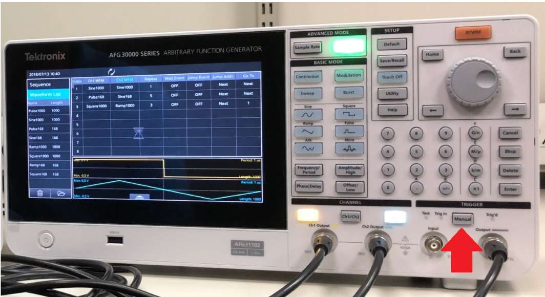
图 109：“手动触发”按钮
