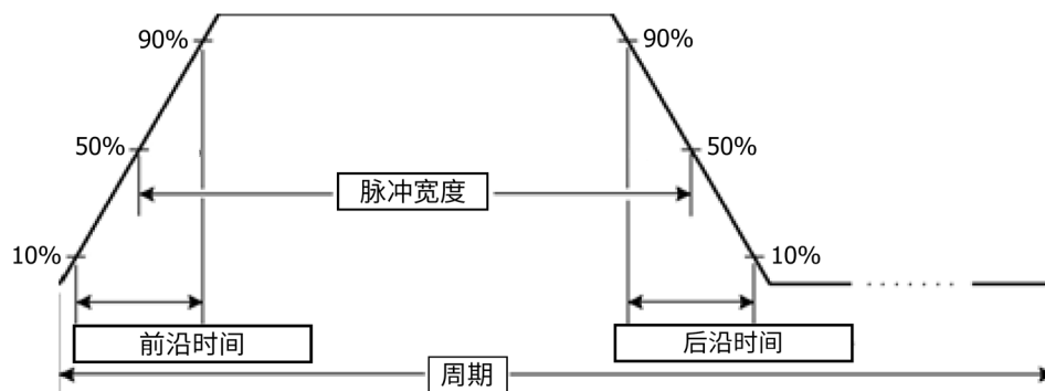
图 28：脉冲周期宽度
