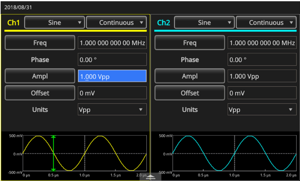
图 7：振幅按钮为有效状态
