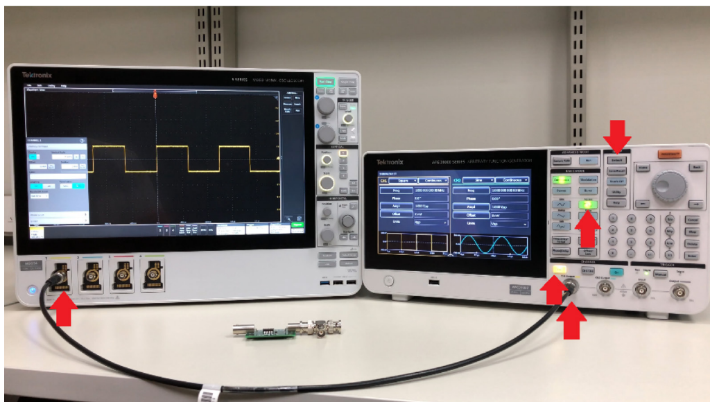
图 63：带连接的 AFG31000 InstaView 设置的概述
