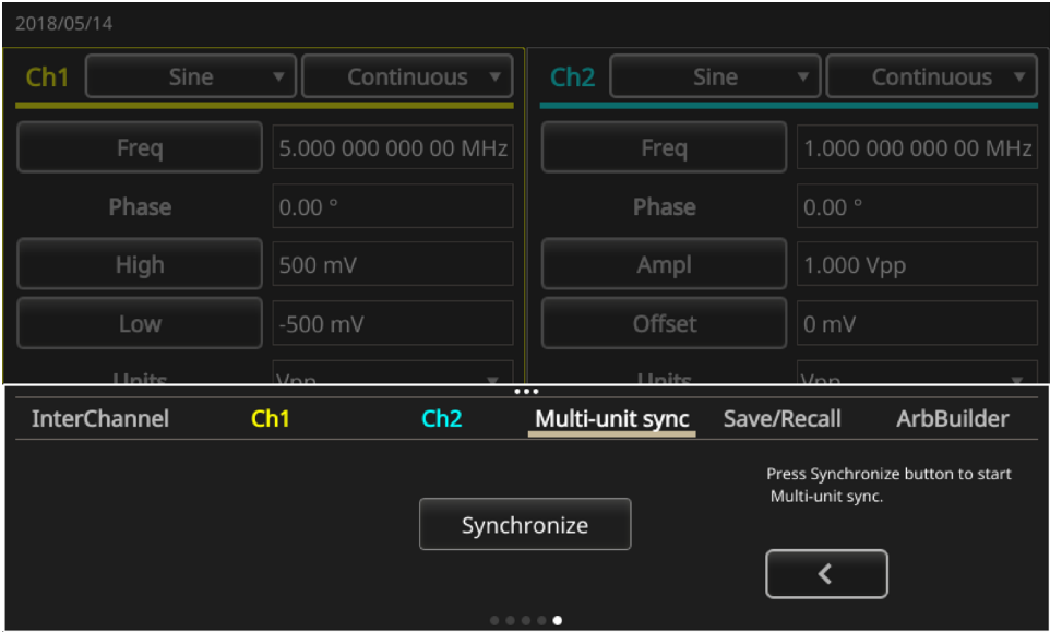
图 58：“多仪器同步” 仪器选项卡 5
