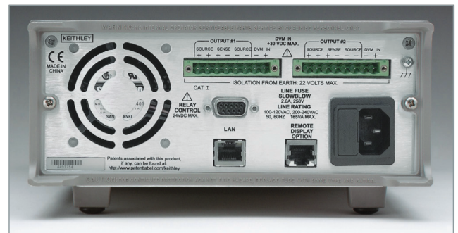
图 9. 2306-LAN 后面板
