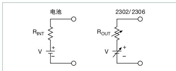
图 1. 电池与 2302/2306 简化示意图
