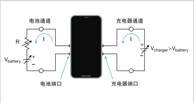
图 6. 对于充电器控制电路测试应用，2306 型和 2306-PJ 型电池 / 充电器模拟器可以提供充电器模拟电源功能以及放电电池模拟器功能。
