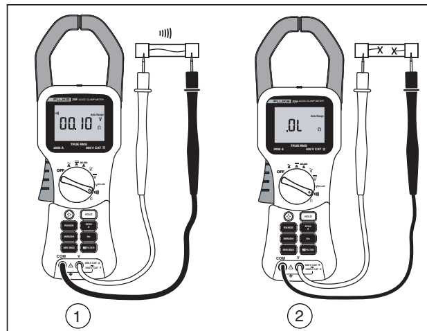
图 7. 测试通断性
