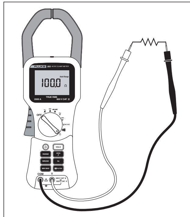
图 8. 测量电阻
