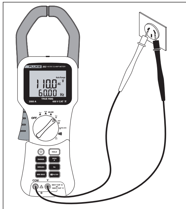
图 5. AC 交流电压测量
