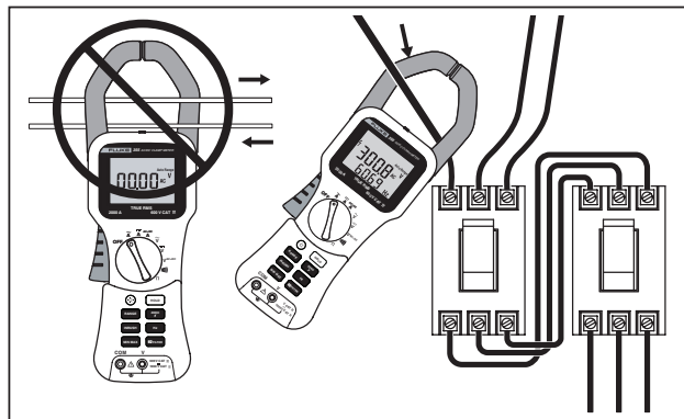
图 3. 连接仪表
