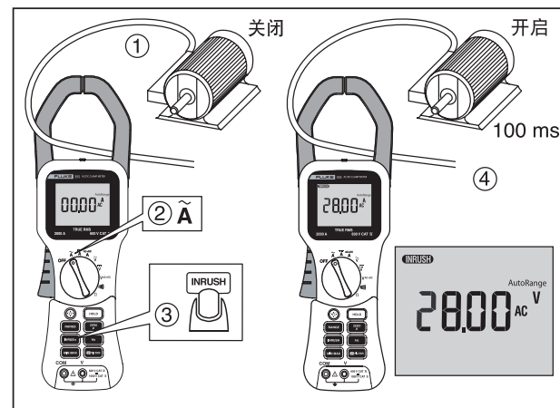
图 4. 测量浪涌电流
