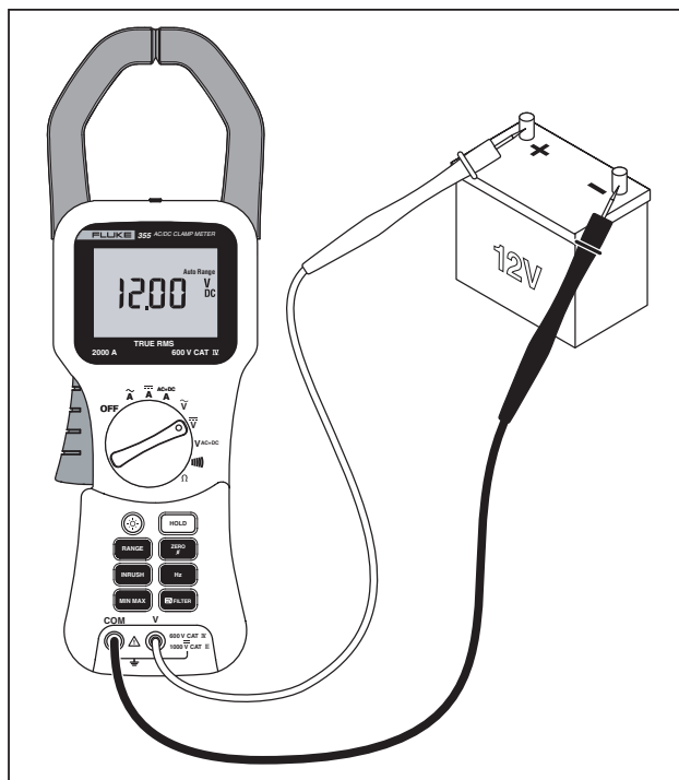
图 6. 直流电压测量
