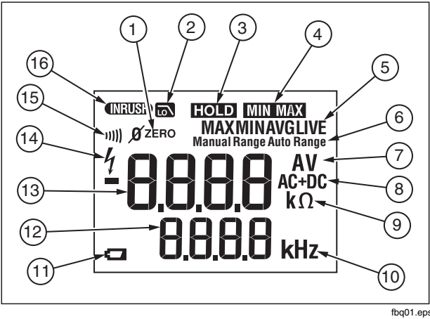
图 2. 显示屏
