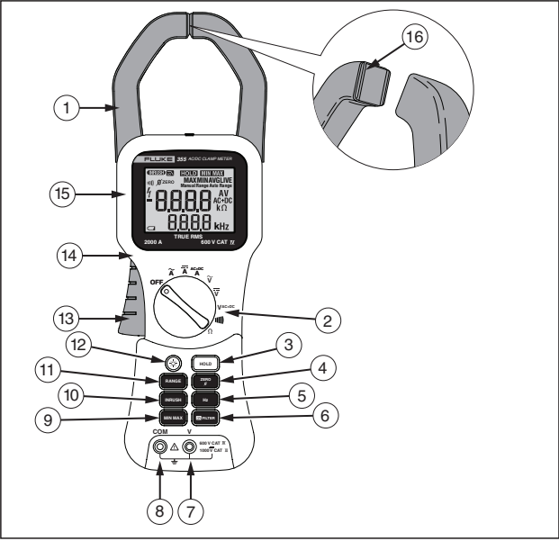
图 1. 特性的位置（显示 355 型）
