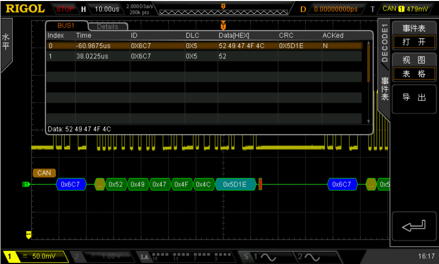
图 8-13 CAN 解码列表（表格）
