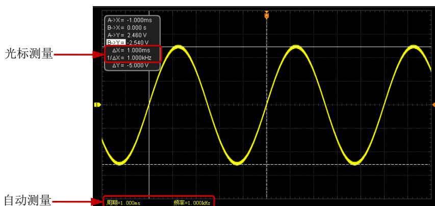
图 6-7 手动光标测量
