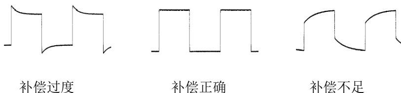
图 1-9 探头补偿
