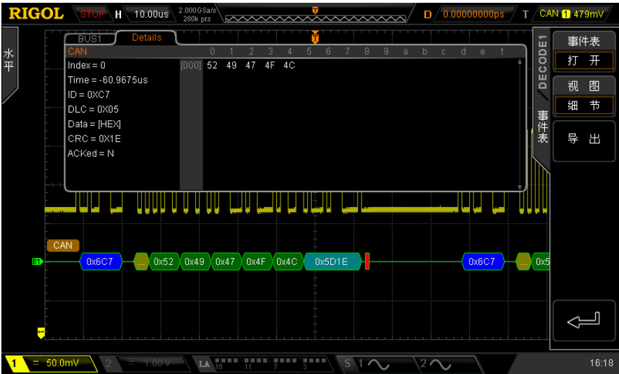
图 8-14 CAN 解码列表（细节）
