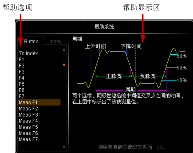
图 1-14 帮助界面
