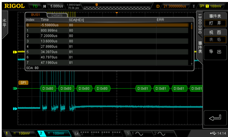
图 8-11 SPI 解码列表
