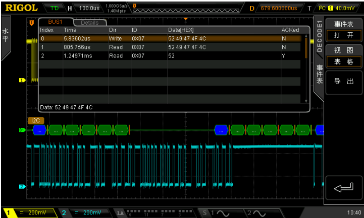
图 8-6 I2C 解码列表（表格）
