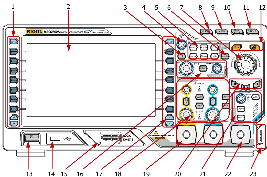
图 1-10 前面板总览
