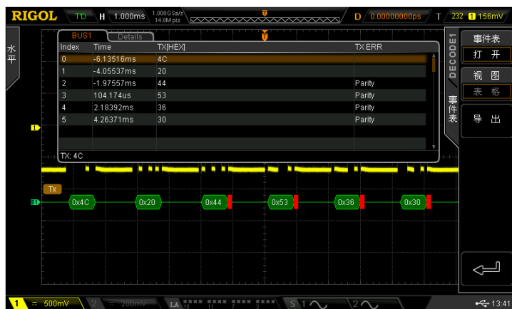
图 8-4 RS232 解码列表
