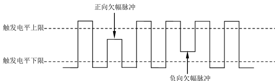
图 5-4 欠幅脉冲
