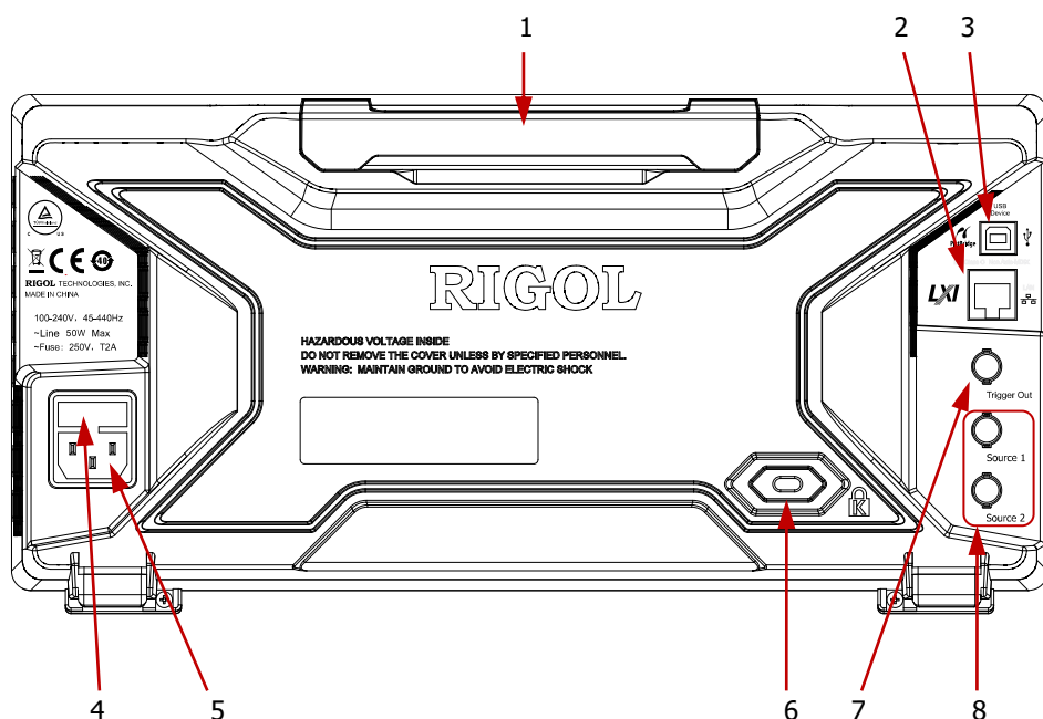
图 1-11 后面板总览
