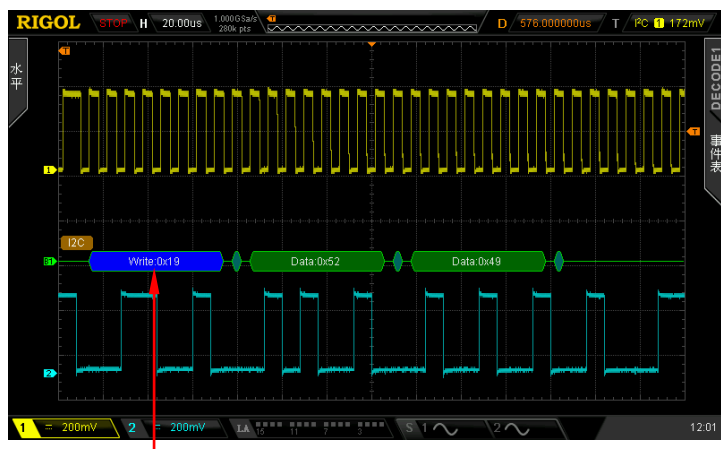
图 8-8 解码时的地址信息示例
