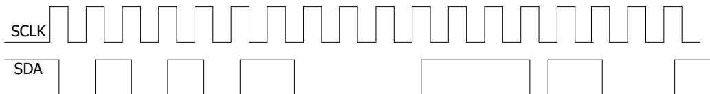
图 8-5 I2C 串行总线
