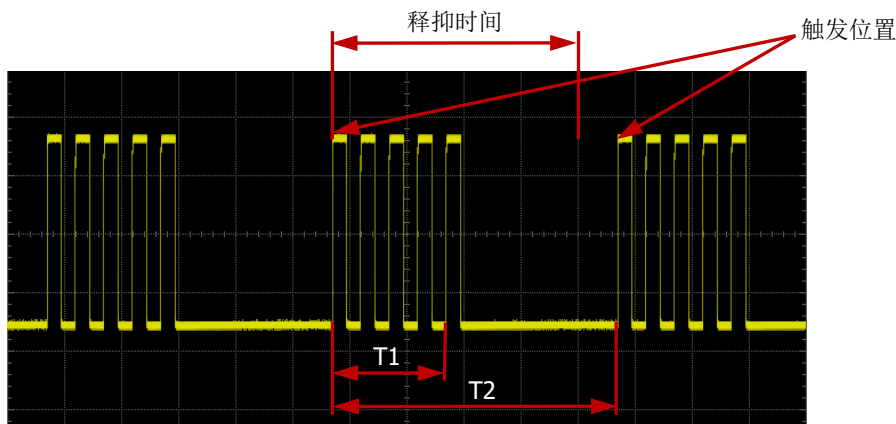
图 5-2 触发释抑示意图
