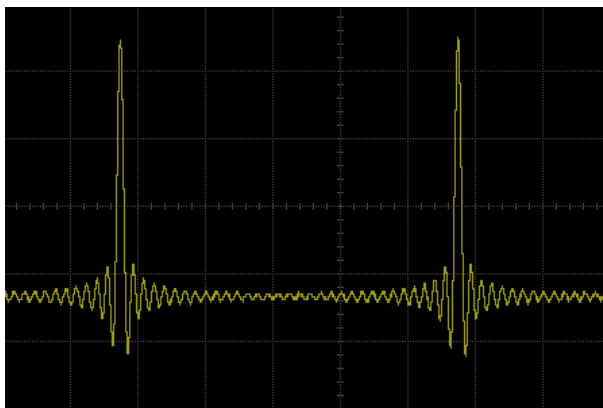
图 13-2 Sinc 函数的波形示意图
