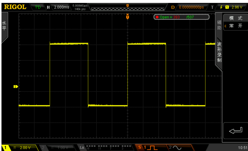
图 11-1 录制常开模式的应用
