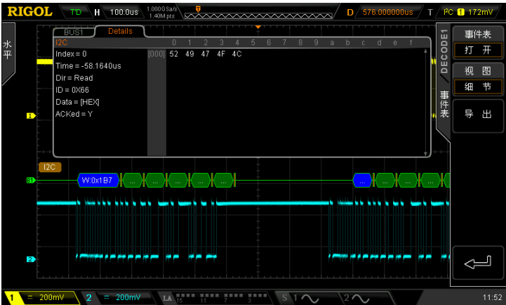
图 8-7 I2C 解码列表（细节）
