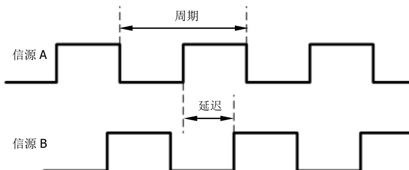
图 6-4 延迟和相位
