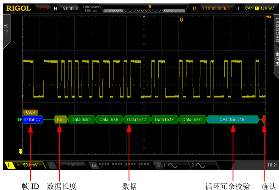
图 8-15 已解码的 CAN 数据示意图
