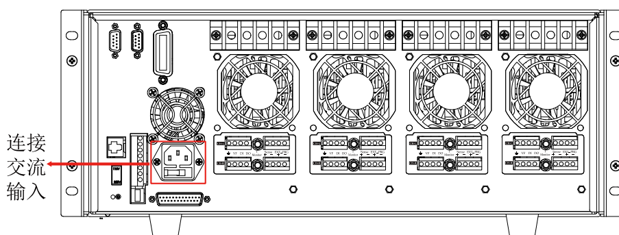
图1-6 连接交流输入图
