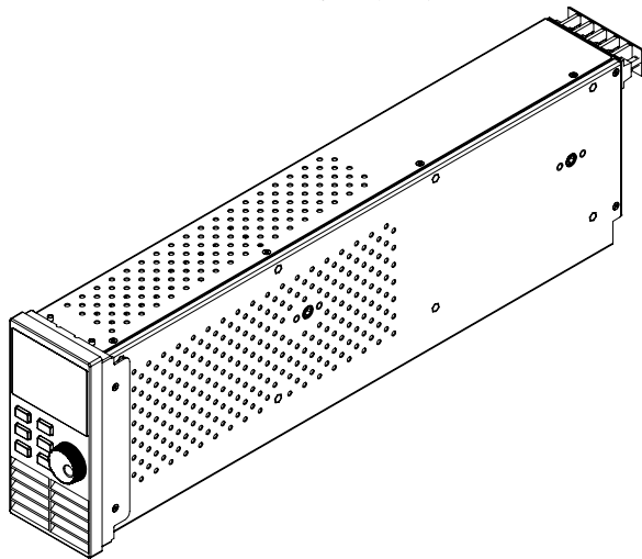
IT8722/IT8723/IT8722B 模组尺寸图
