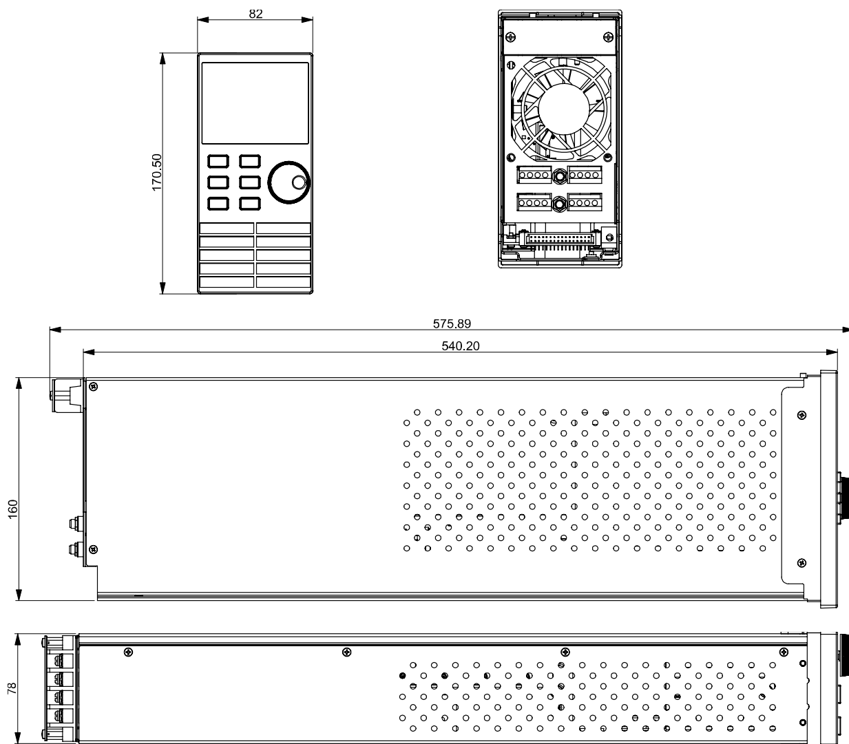
详细尺寸图
