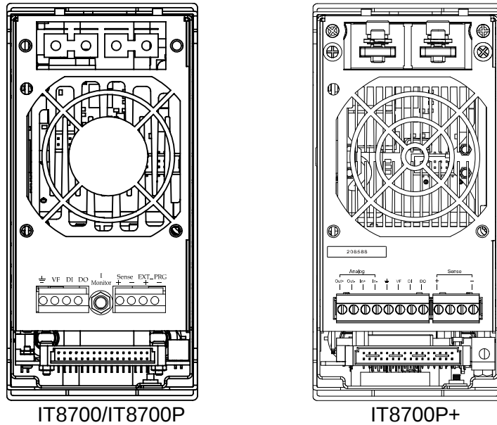
图 3-9 单路模组后面板端子功能
