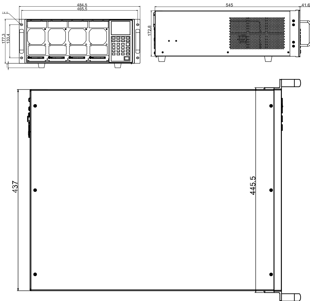
详细尺寸图
