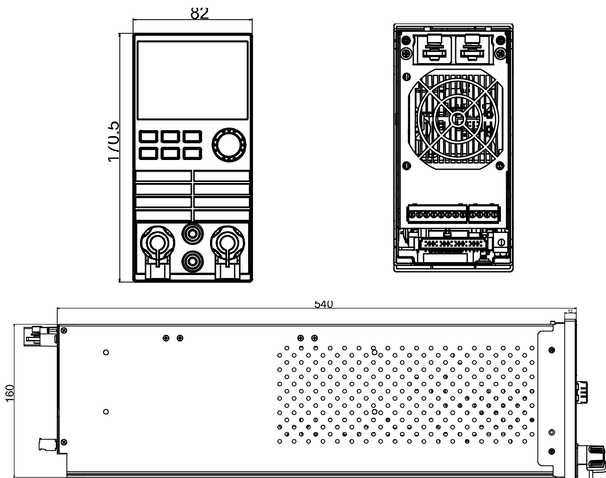
详细尺寸图
