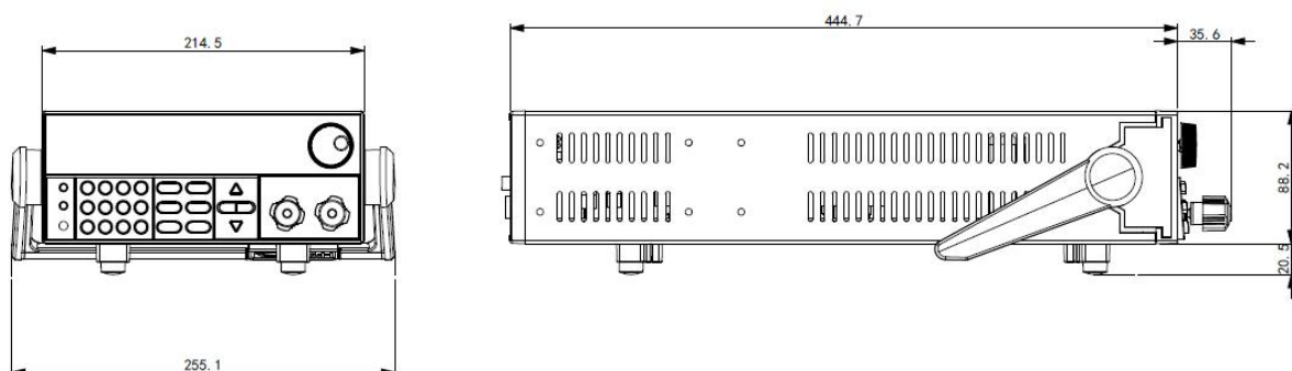
详细尺寸图
