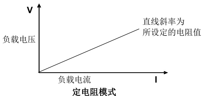
图3-2 CR模式电压电流关系图
