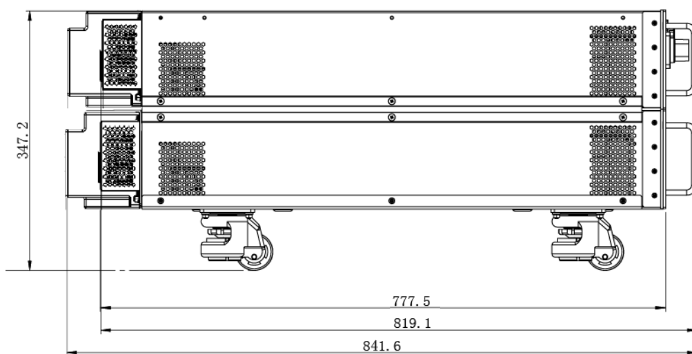
IT7863E-350-270 机型
