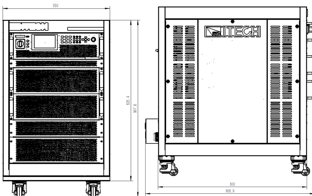
IT7863E-350-270 机型
