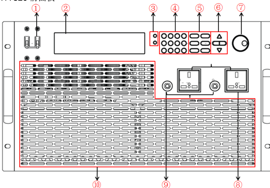
IT7326 前面板
