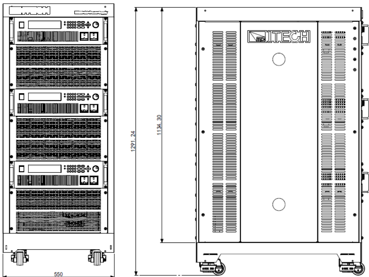
详细尺寸图
