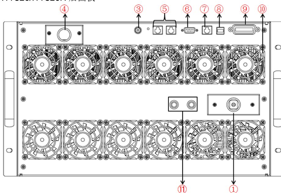
IT7326/IT7326H 后面板
