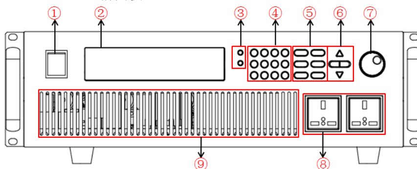
IT7322/IT7324 前面板
