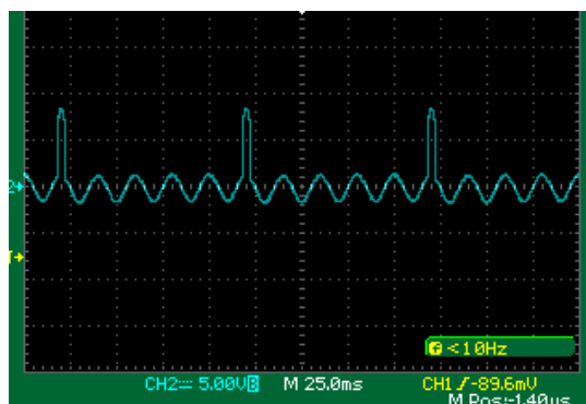
突波波形
