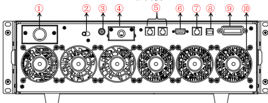
IT7322/IT7322H/IT7324/IT7324H 后面板
