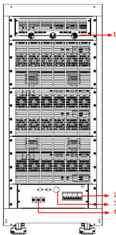
IT7326HT 后面板图示
