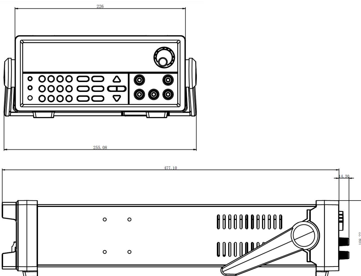
详细尺寸图
