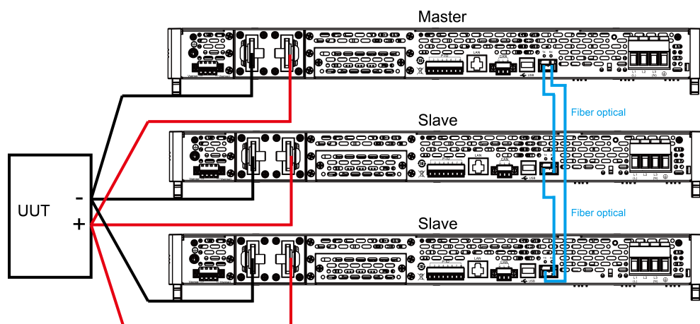
图 5-1 线路连接图
