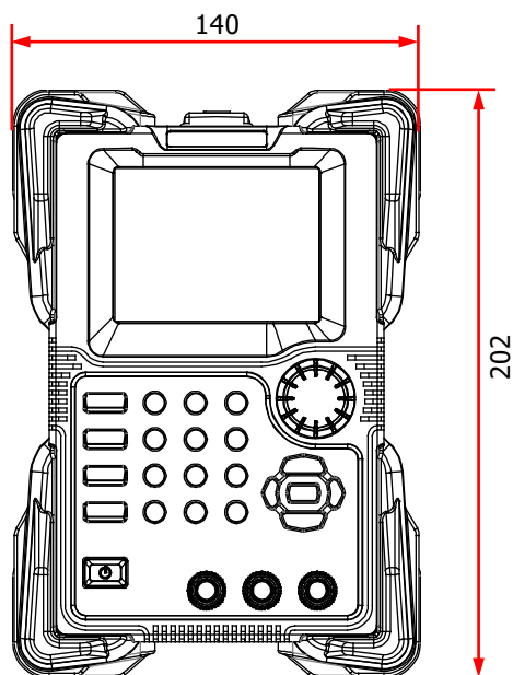
图 1-1 正视图
