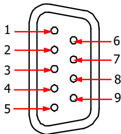
图 2-6 RS232 接口
