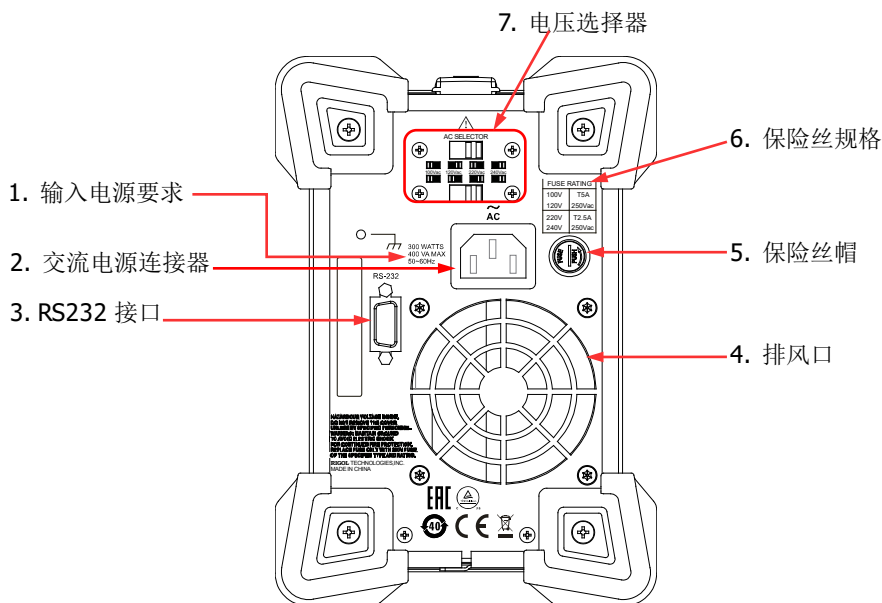
图 1-4 后面板
