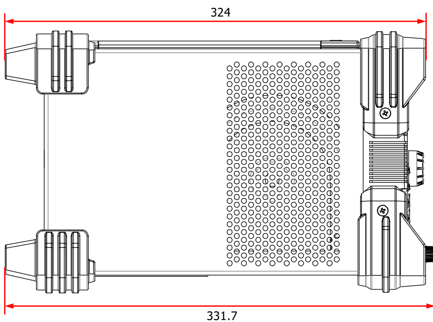
图 1-2 侧视图
