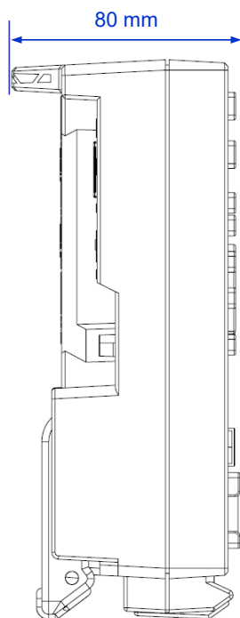
图 4.2 侧视图
