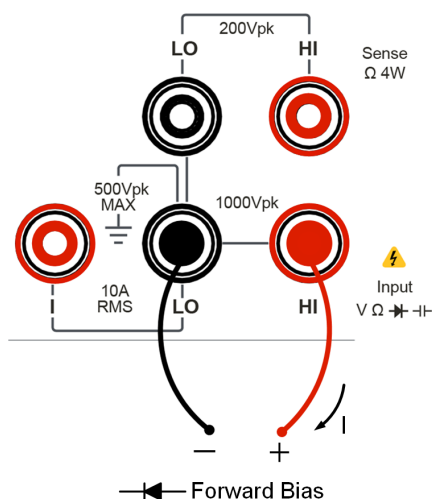
图 5.27 二极管检测示意图
