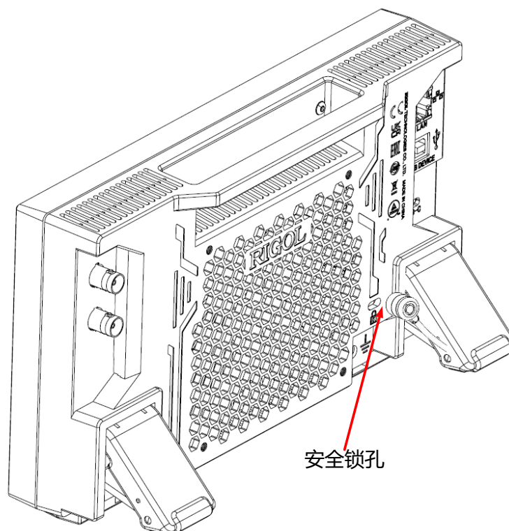
图 4.14 使用安全锁
