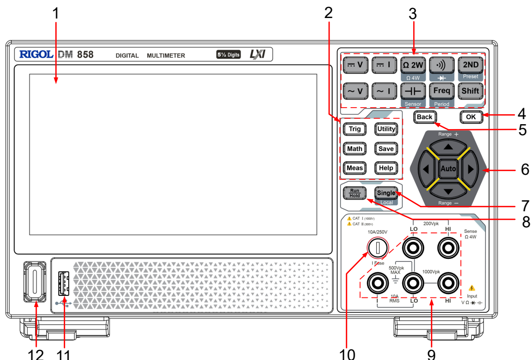
图 4.5 DM858 前面板
