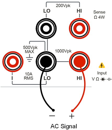
图 5.32 周期测量连接示意图
