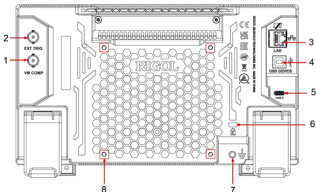
图 4.6 后面板
