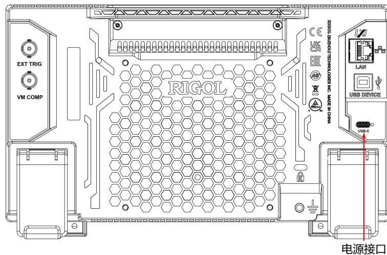
图 4.4 连接电源
