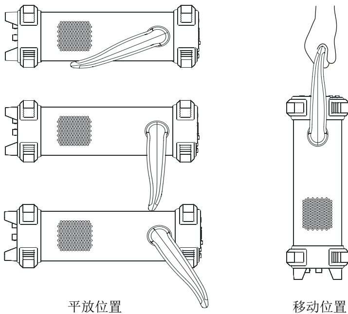
图 1-2 放置仪器
