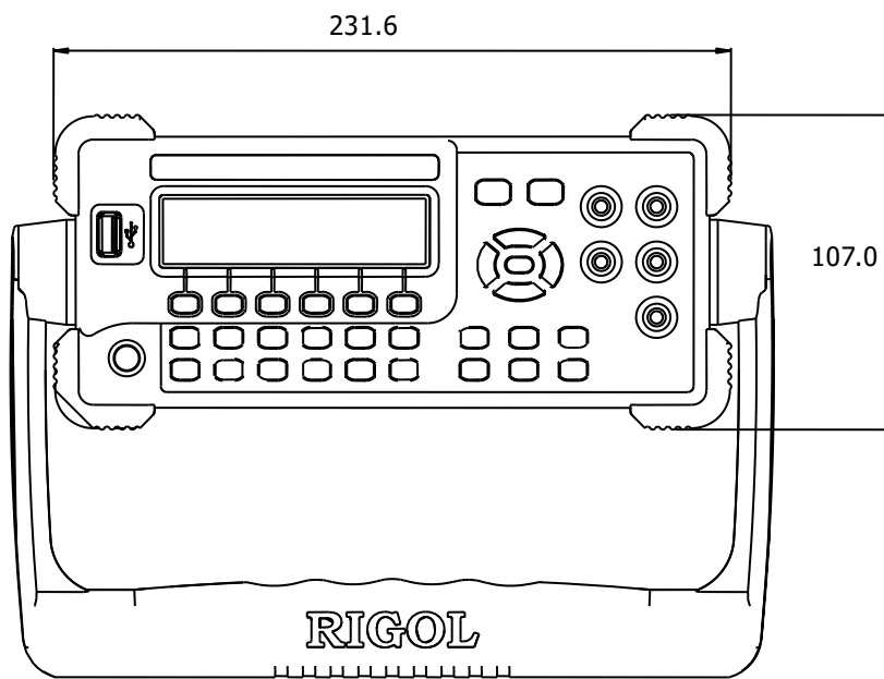
图 1-3 正视图
