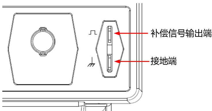
图 5.4 补偿信号
