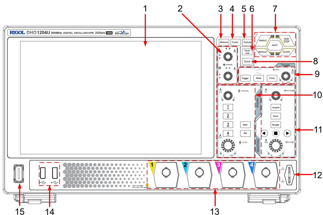
图 4.1 前面板（4 通道）
