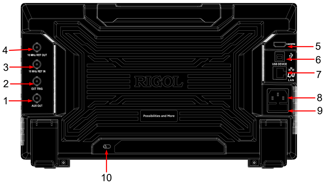
图 4.3 后面板
