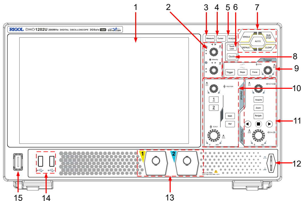
图 4.2 前面板 (2 通道)
