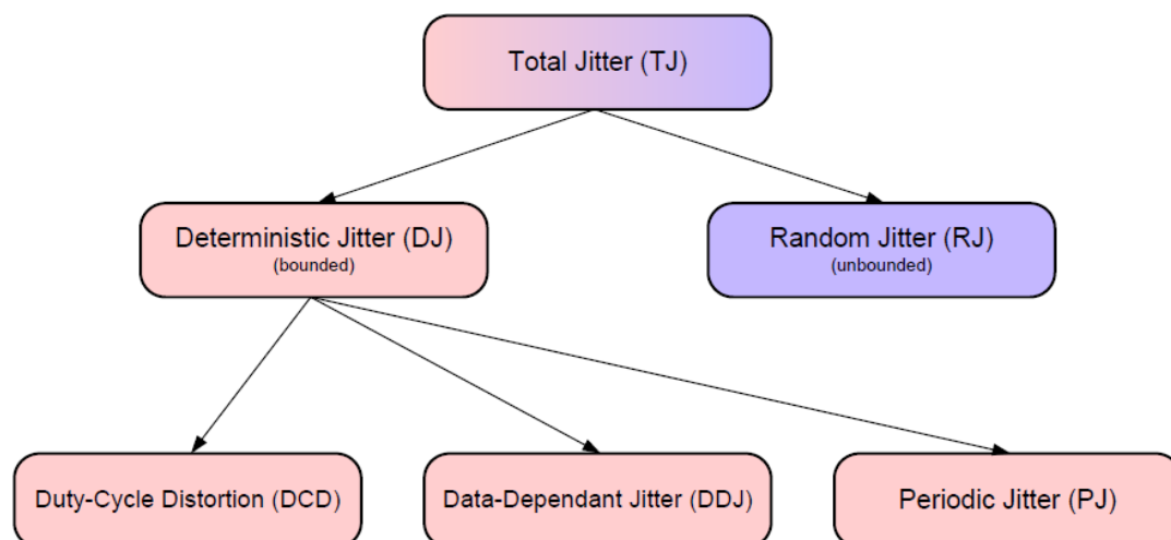
图 31.1 抖动的分解
