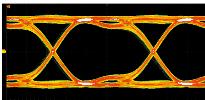
使用750 MHz带宽和1.5 GHz带宽分别对1 Gb/s信号进行眼图观测
