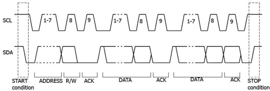
图 3.9 I2C 帧格式示意图
