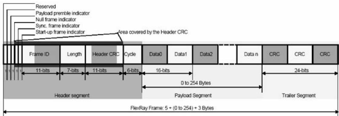
图 3.14 FlexRay 总线帧格式
