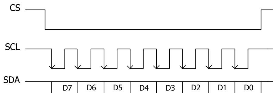
图 3.10 SPI 总线时序图
