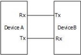
图 3.2 RS232 串行总线示意图
