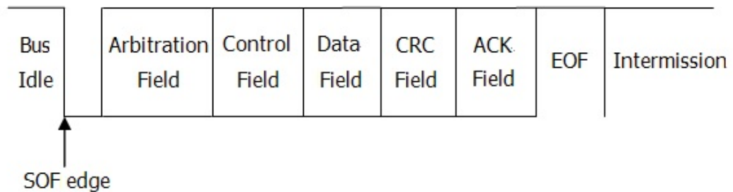
图 3.11 CAN 总线数据帧格式
