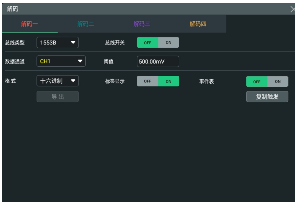
图 17.24 1553B 解码菜单
