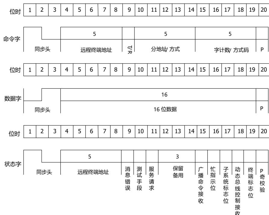
图 8.42 1553B 总线命令字、数据字和状态字格式图
