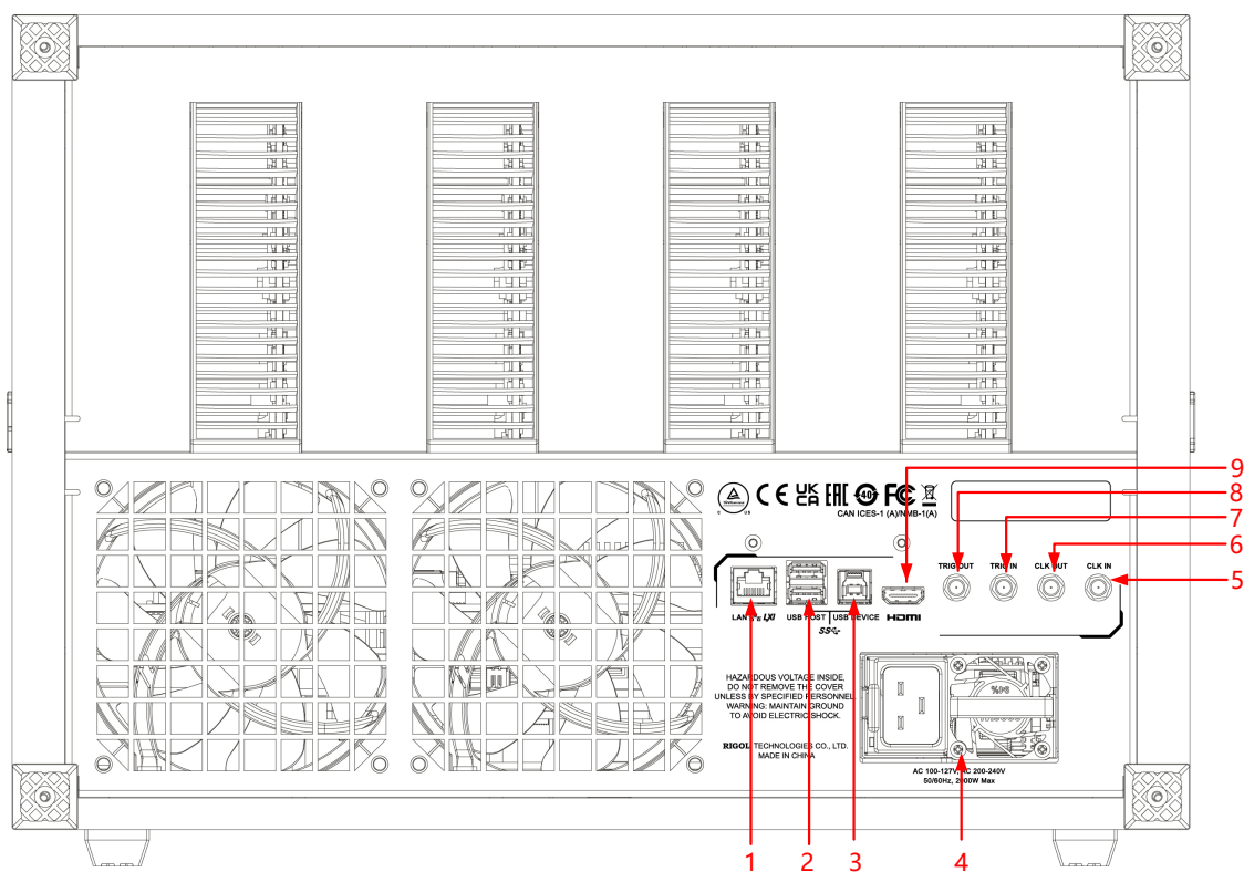
图 4.11 DS80000 后面板
