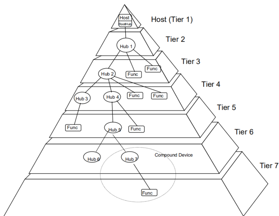
图 17.26 USB 拓扑图
