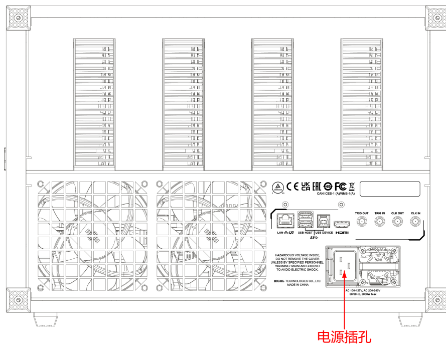
图 4.3 连接电源
