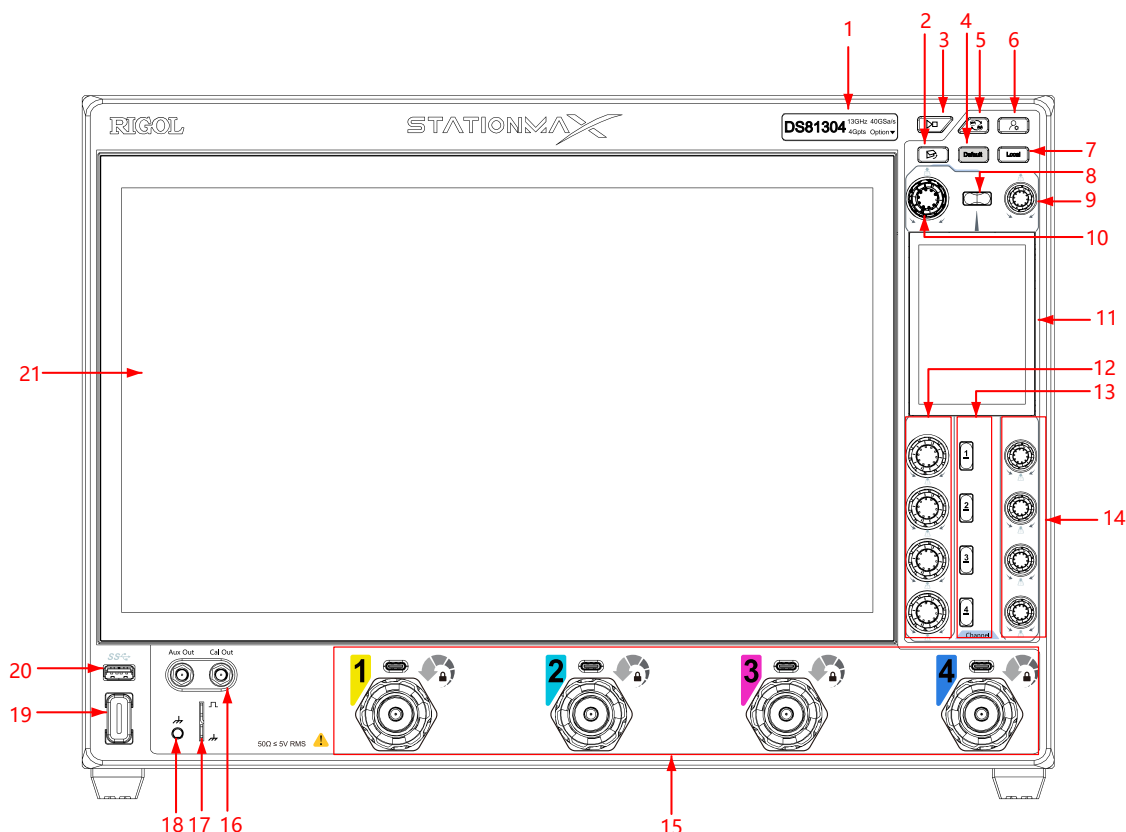
图 4.10 DS80000 前面板
