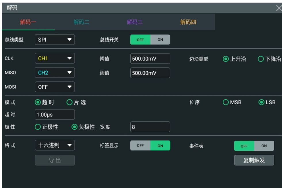
图 17.12 SPI 解码菜单
