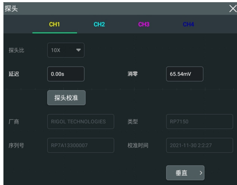
图 5.4 RP7000 系列、PVA7000 系列或 PVA8000 系列探头设置菜单
