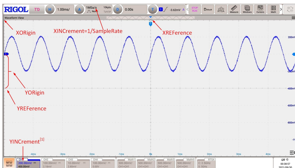
图 3.17 RAW 模式下的参数定义
