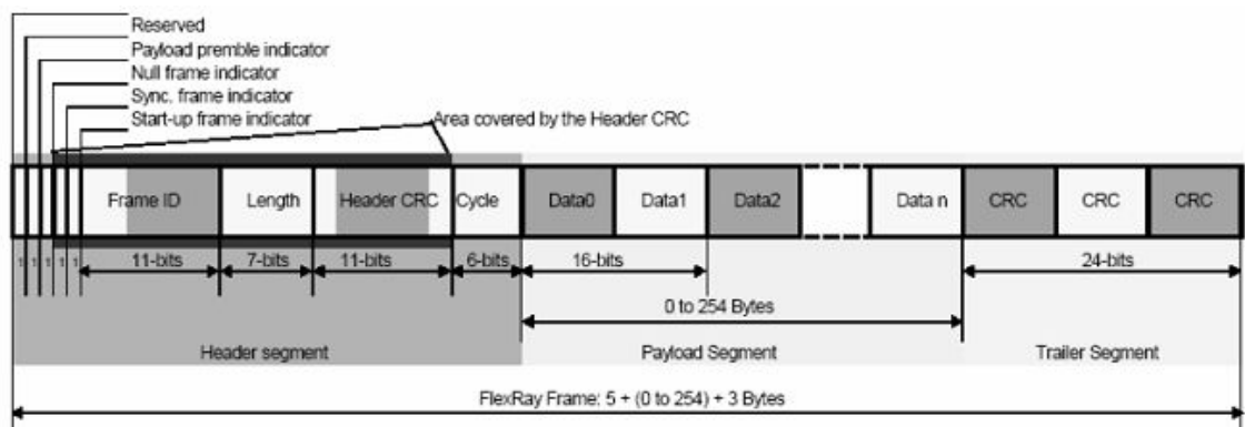
图 3.12 FlexRay 总线帧格式
