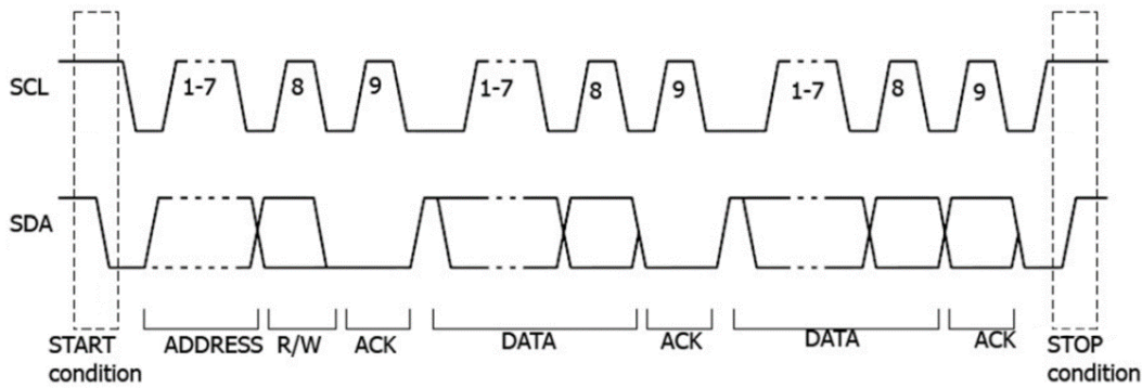
图 3.9 I2C 协议示意图
