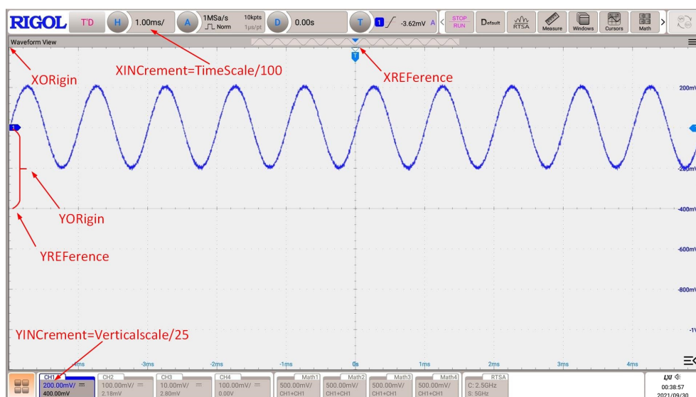
图 3.16 NORMAL 模式下的参数定义
