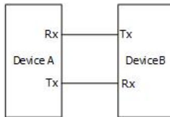
图 3.2 RS232 串行总线示意图
