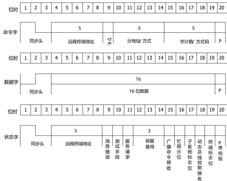
图 3.15 1553B 总线命令字、数据字和状态字格式图
