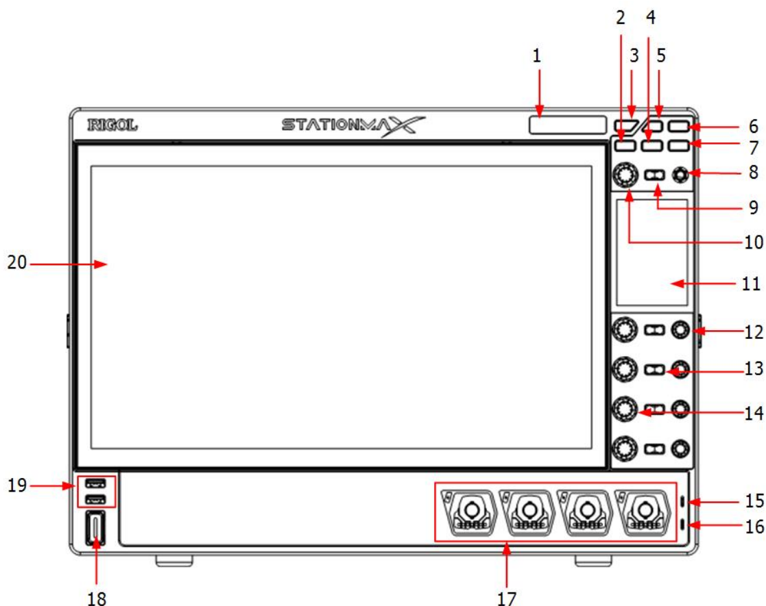
图 4.1 前面板
