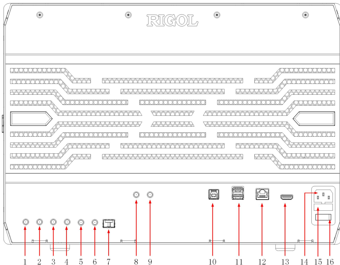
图 4.2 后面板
