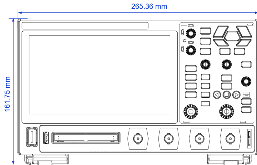
图 4.1 正视图
