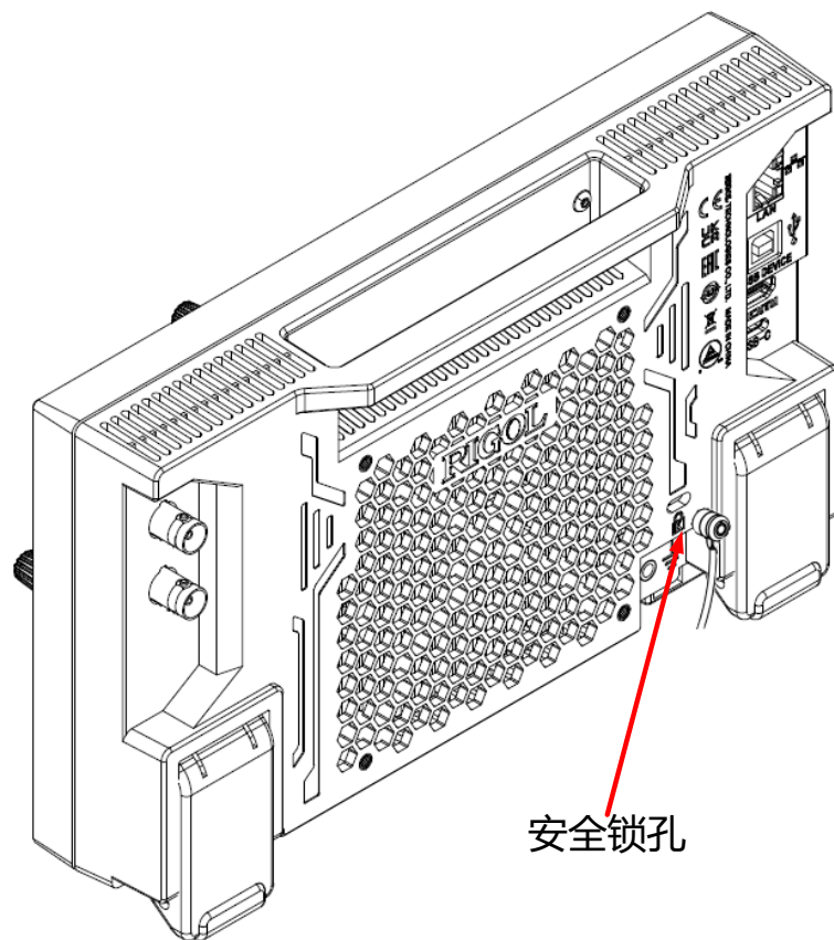
图 4.20 使用安全锁
