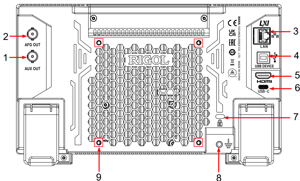
图 4.11 后面板
