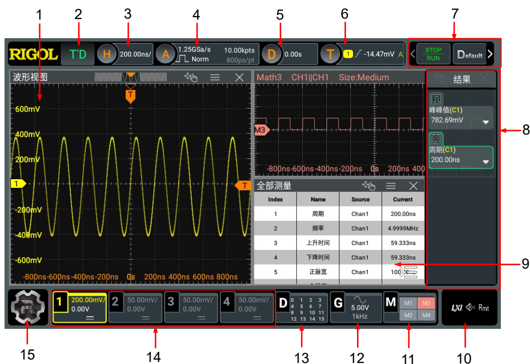
图 4.12 用户界面
