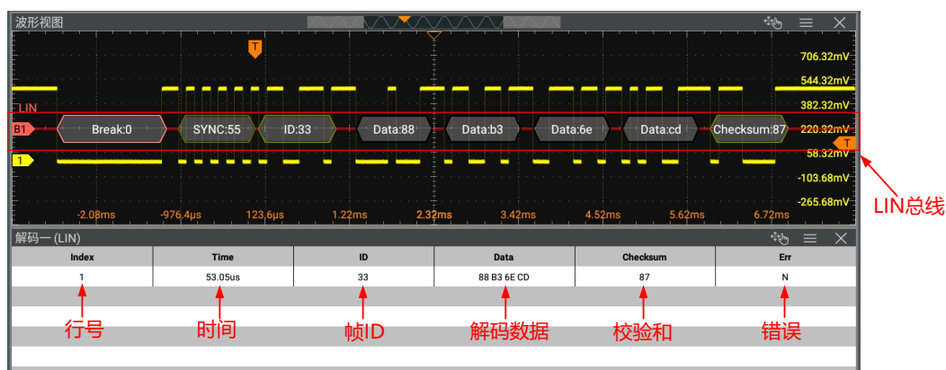
图 18.14 LIN 解码事件表
