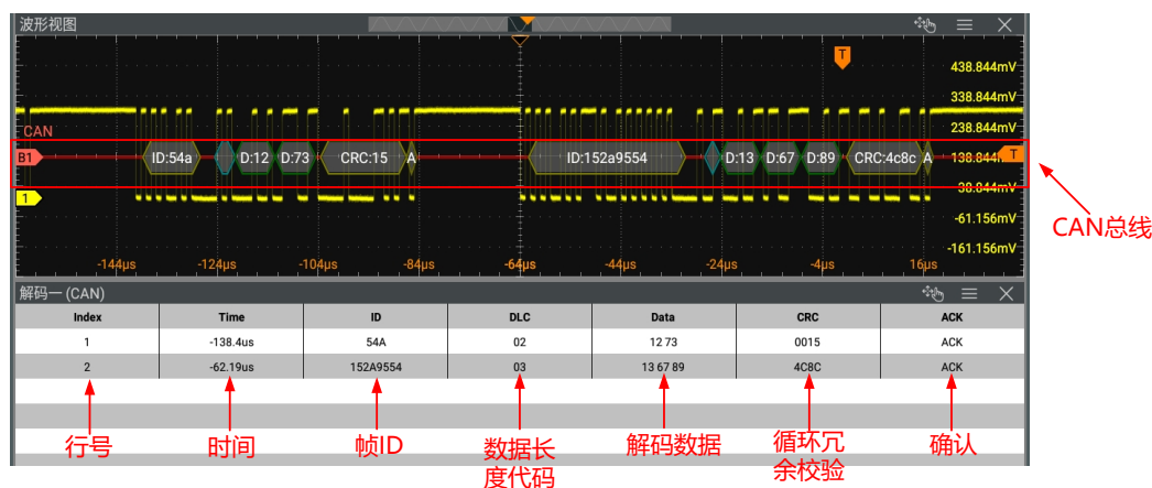
图 18.17 CAN 解码事件表
