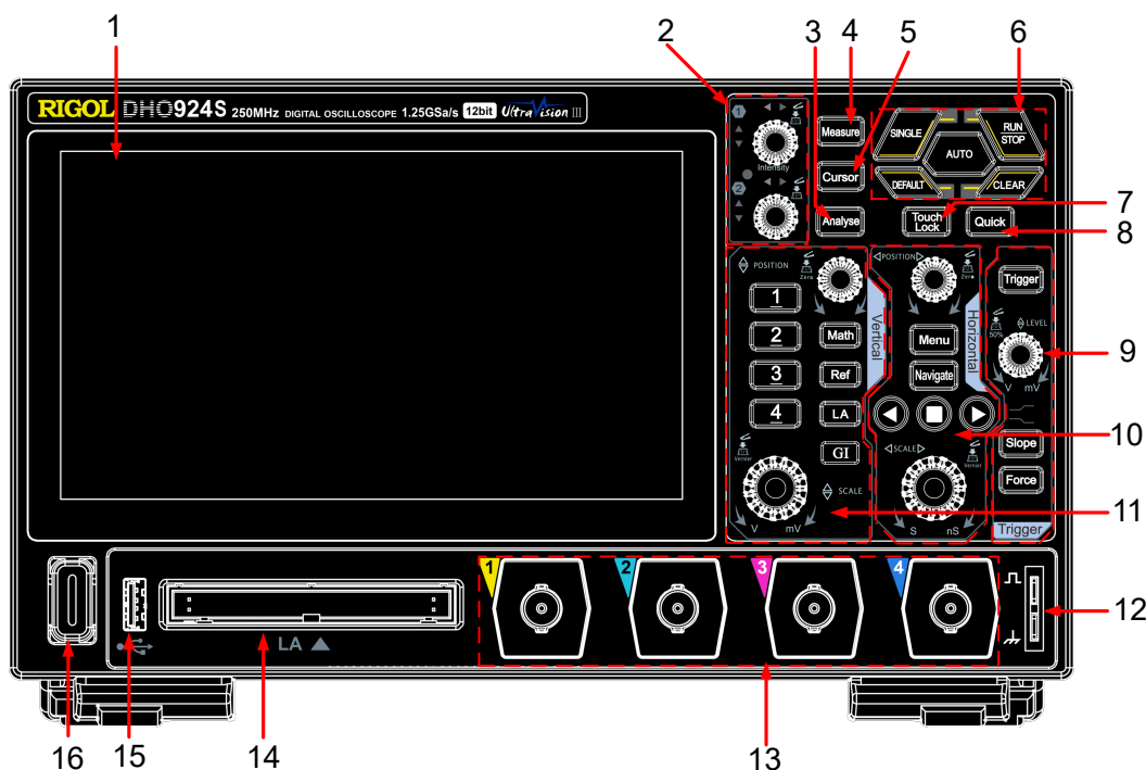
图 4.10 前面板
