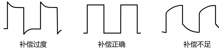
图 4.8 探头补偿
