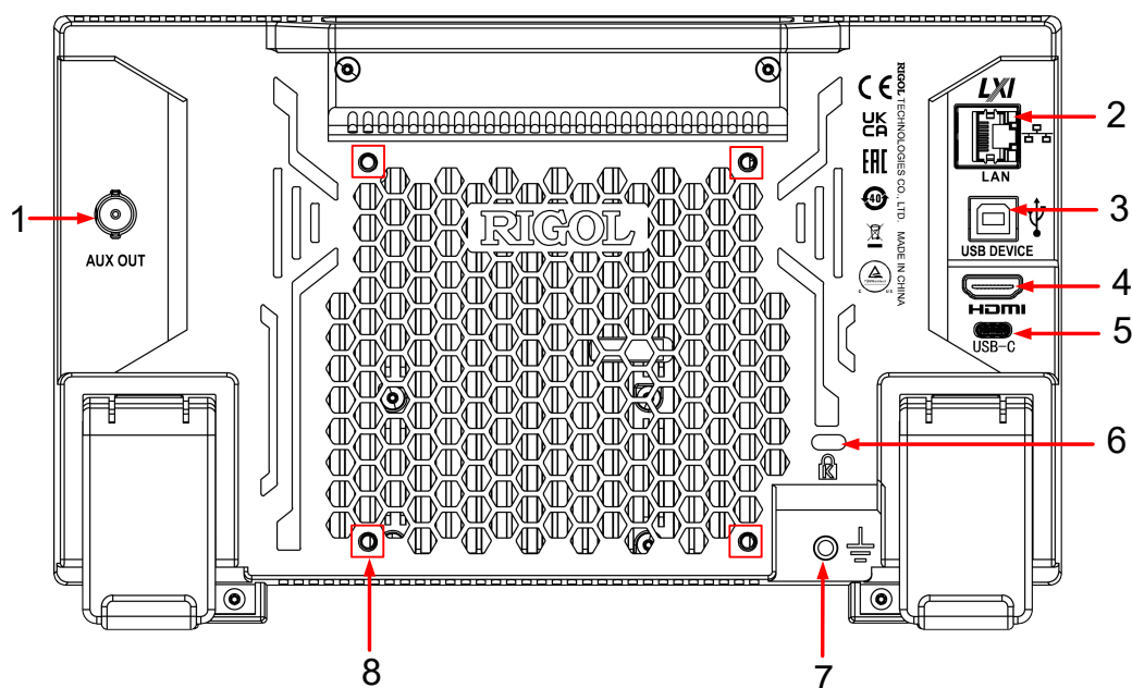
图 4.11 后面板
