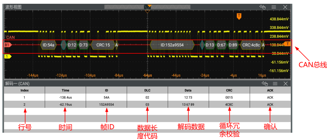
图 15.15 CAN 解码事件表
